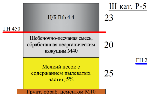
Рис. 2.3. Конструкции дорожных одежд в Мурманской области
