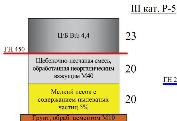
Рис. 2.15. Конструкции дорожных одежд в Самарской области
