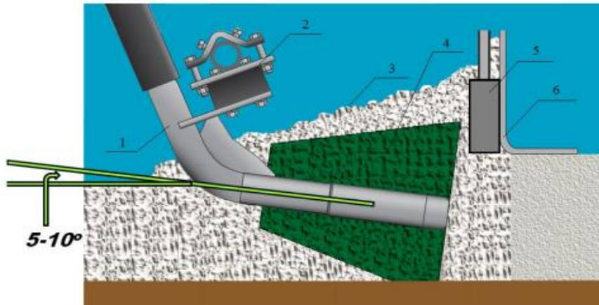
1 – глубинный вибратор; 2 – крепление вибратора на бетоноукладчике; 3 – бетонная смесь; 4 – этюра амплитуды колебаний по длине вибратора; 5 – трамбующий брус укладчика; 6 – формирующая плита укладчика
