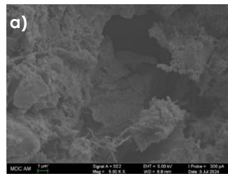
Микроструктура сколов образцов а) цементогрунта без модификаторов, б) цементогрунта с комплексным модификатором
