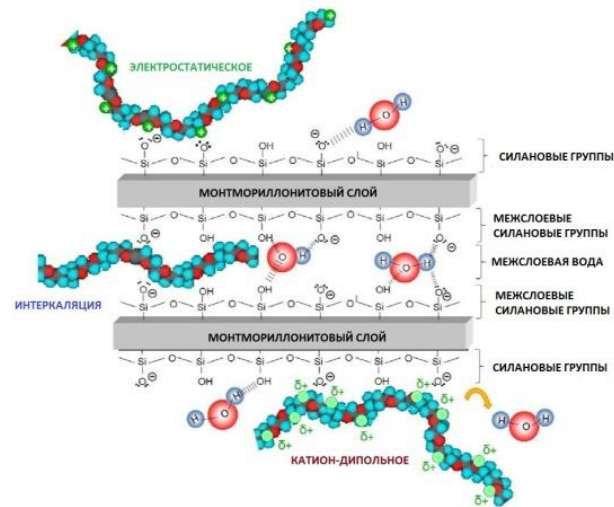
Взаимодействие полиэтиленгликоля с алюмосиликатными слоями монтмориллонита
