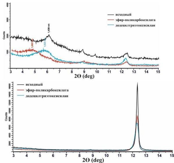
Рисунок 1 – Дифрактограммы исследуемых глин: — не модифицированная глина; — глина, модифицированная эфиром поликарбоксилата; — глина, модифицированная додецилтриэтоксисилоном 1 – монтмориллионовая глина; 2 – каолиниевая глина
