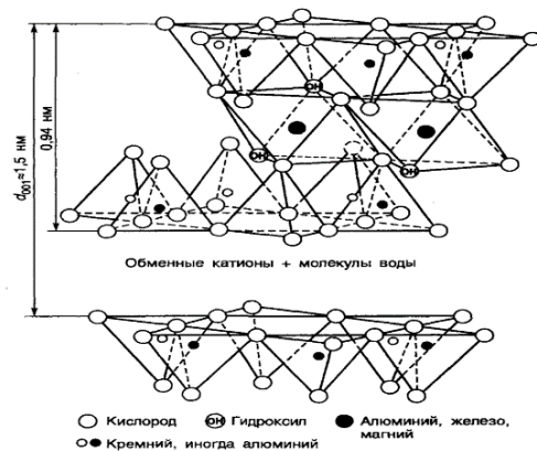
Структура монтмориллонита
