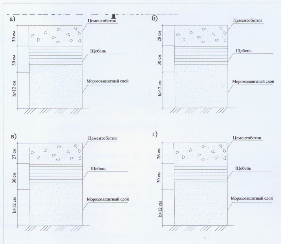
Рис. 2. Конструкции дорожных одежд с цементобетонным покрытием на основании из щебня, применяемые в Германии при приведенной нагрузке эквивалентной 10-тонным осевым проездам:
